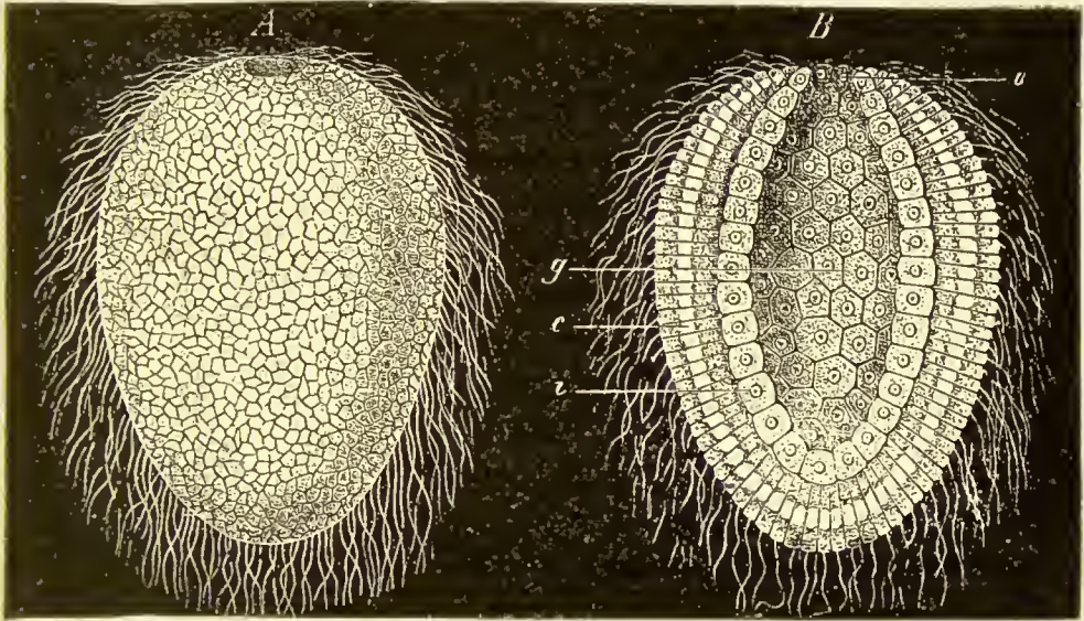
GASTRULA (OLYNTHUS.)
